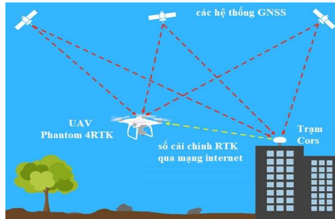
Hình Phương pháp định vị tâm chụp cho UAV bằng Network RTK (nguồn: Escadrone.com, 2020).
