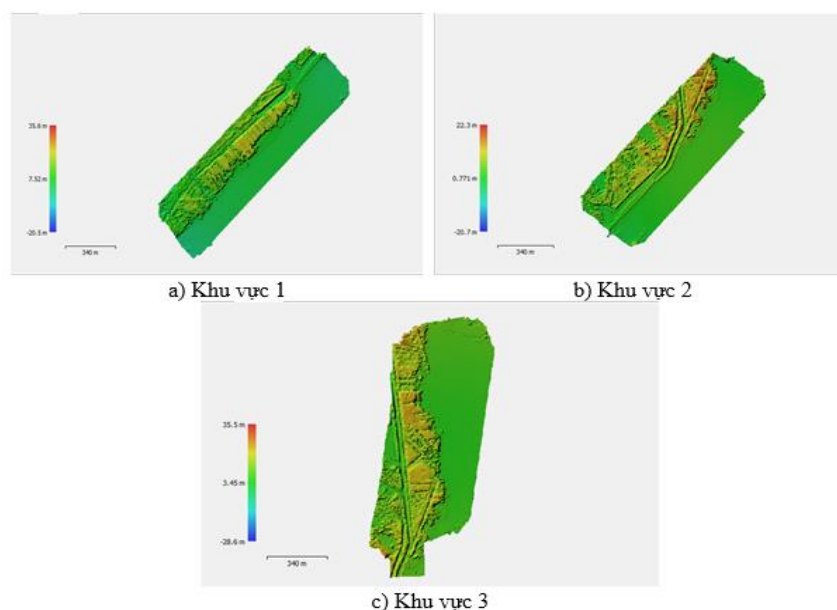
Hình 3: Kết quả tạo ảnh Orthomosaic chia theo 3 tiểu khu vực.
