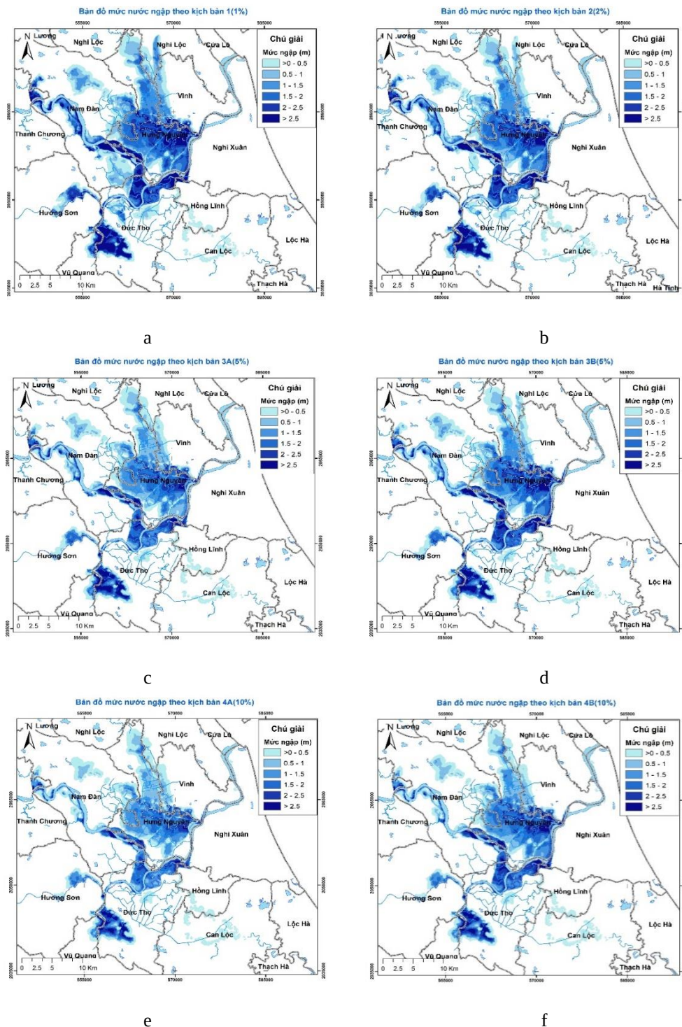
Hình 4. Kết quả các kịch bản lũ từ mô hình thủy lực(a,b,c,d,e,f tương ứng với các kịch bản 1,2,3A,3B, 4A, 4B,) theo dữ liệu năm 2017.
