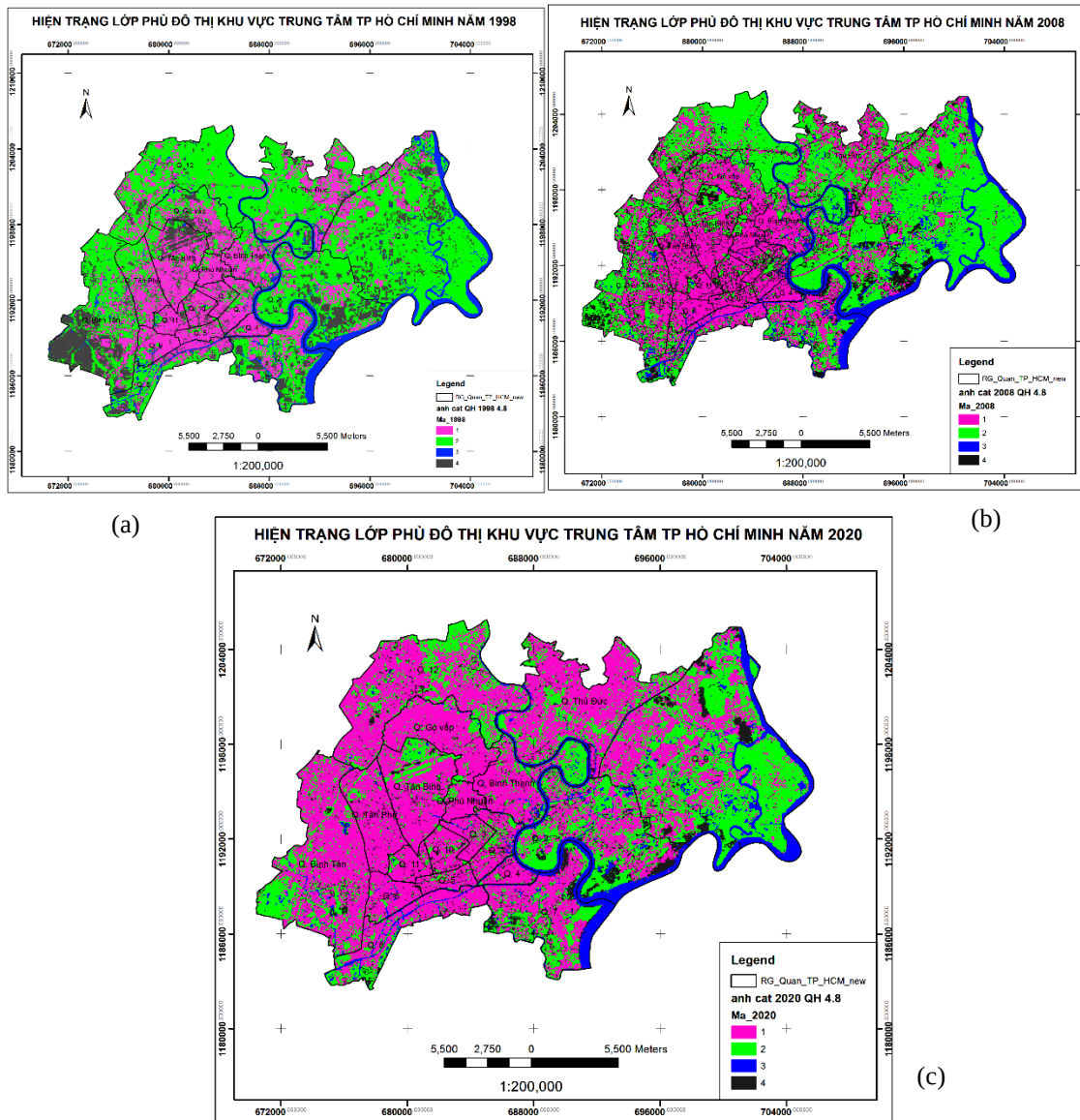
Hình 3: Hiện trạng lớp phủ đô thị khu vực trung tâm TP Hồ Chí Minh năm 1998 (a), 2008 (b), 2020 (c) Trong đó: 1 - Bề mặt không thấm; 2 - Thực vật; 3 - Mặt nước; 4 - Đất trống.
