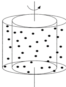
Hình Cặp hình trụ miêu tả SfM (C. Caudek and N. Rubin, 2001)
